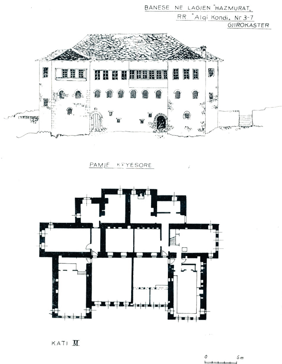
Fig. 3 Maison double de Gjirokastra, Albanie (d'après Emin Riza). Façade et plan du deuxième niveau ; dans E. Riza, « Banesa dyfamiare në qytet », p. 119, planche I, maison n° 3.
