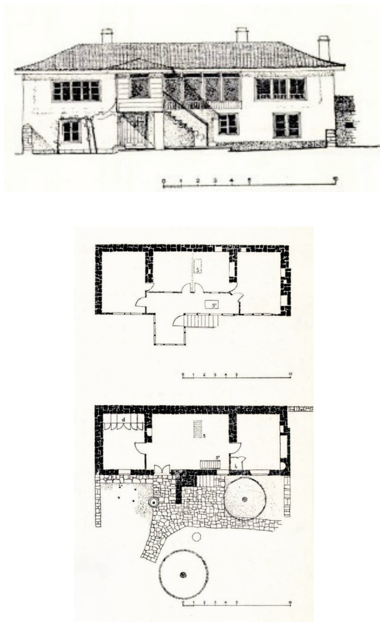
Fig. 27 Maison double de Mangalia – Dobroudja, Roumanie (d'après arch. Gheorghe Petrașcu) ; dans Gh. Petrașcu « Pe urmele unei arhitecturi populare valoroase », Arhitectura R.P.R. 9, 1956, p. 26, maison C.
