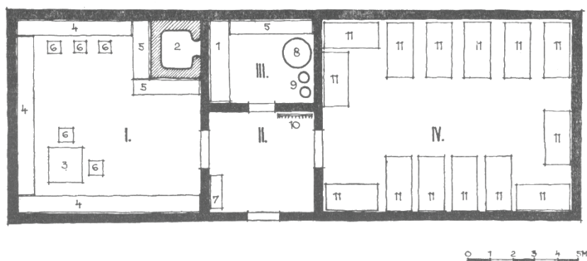
Fig. 19 Maison slovaque du département de Zvolen (d'après Jan Botík) ; I – chambre habitée ; II – chambre de passage ; III – chambre noire ; IV – chambre à dormir ; dans J. Botík, « Rodina ako determinujúci činiteľ foriem obydlia », Lidová stavební kultura (Brno) 7, 1981 [= Lidová stavební kultura v československých Karpatech a přilehlých územích , éd. V. Frolec], p. 160, fig. 76.
