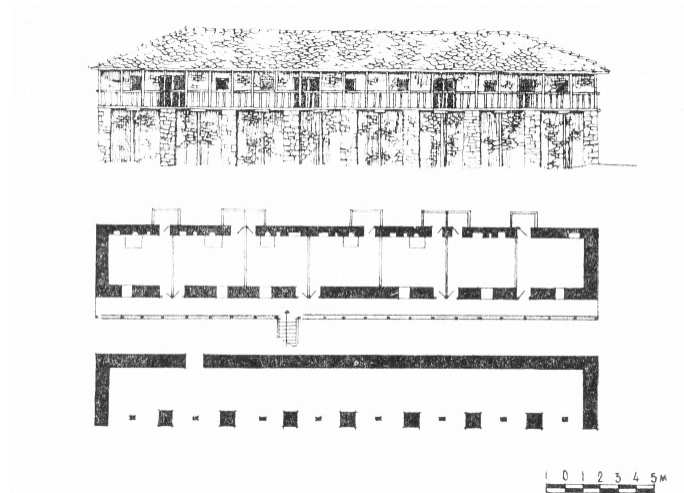
Fig. 9b Maison fortifiée à foyer central, et chambres à dormir, au village de Petit Shëngjin [alb. Shëngjini i Vogël] (d'après Ali Muka). Le plan des chambres à dormir (2) ; dans A. Muka, « L'habitation rurale dans la Malessie... », p. 252, planche IX-1.
