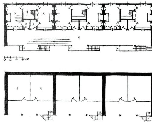
Fig. 16 Maison triple bulgare, Yakoruda (d'après Georgi Kozhukarov). Dans G. Kozhuharov, « Narodnata kŭshta... », p. 74, fig. 48.
