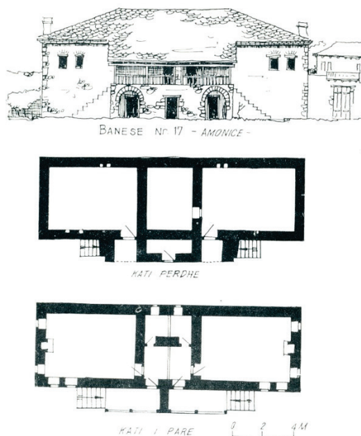
Fig. 1a Maison doubles du village d'Amonicë, Albanie (d'après Emin Riza) ; dans E. Riza, « Banesa popullore në fshatrat e rrethit të Vlorës », Monumentet 15–16, 1978, p. 210, planche VII, maison n° 17.
