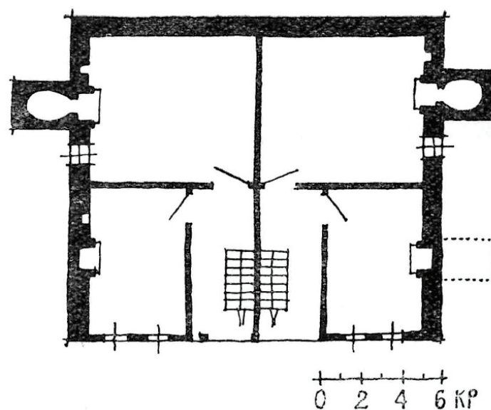
Fig. 14 Maison double bulgare de la région de Pirin (d'après Georgi Kozhuharov) ; dans G. Kozhuharov, « Narodnata kŭshhta v dolinite na rekite Struma i Mesta prez vtorata polovina na XIX v. », Izvestiya na sektsiyata za teoriya i istoriya na gradoustroĭstvo arkhitektura (Sofia), 19, 1966, p. 52, fig. 24.
