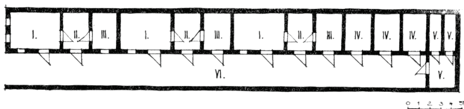
Fig. 22 Maison longue du département de Banská Bystrica : sous un seul toit il y a trois maisons identiques (chambre habitée, pièce de passage, cellier), trois granges et trois étables. La cour longue est parallèle avec la construction (d'après Jan Botík). Dans J. Botík, « Rodina... », p. 181, fig. 86.
