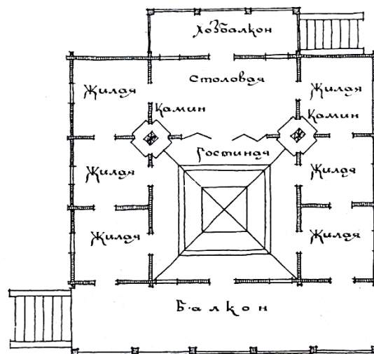
Fig. 24 Maison géorgienne à six chambres à habiter ( zhilaya ), deux foyers ( kamin ), une chambre d'hôtes ( gostinaya ), et une chambre à manger ( stolovaya ) (d'après Mihail Garakanidze – les noms des chambres sont donnés en russe) ; dans M. Garakanidze, Gruzinskoe dereviannoe zodgestvo , planche 40 – maison type 5.
