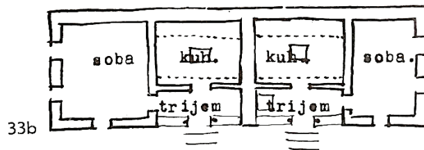
Fig. 15 Maison double croate de Golobrdac (d'après Aleksandar Freudenreich) ; dans A. Freudenreich, Kako narod gradi , Zagreb, 1972, p. 32, fig. 33a et 33b.
