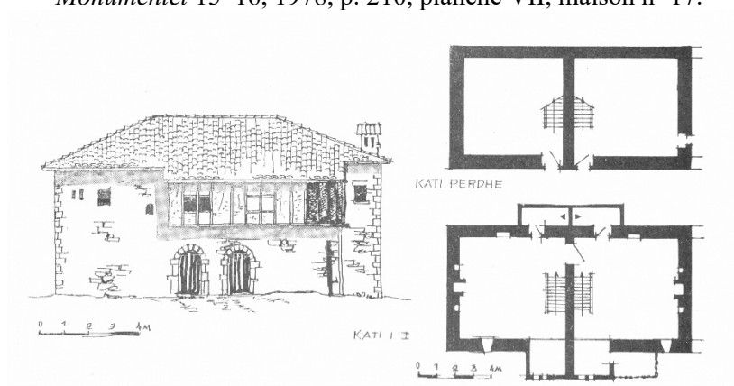
Fig. 1b Maison double du village de Shpërdhet, Albanie (d'après Pirro Thomo) ; dans P. Thomo, Banesa fshatare e Shqipërisë veriore , Tirana, 1981, p. 160, fig. 36.
