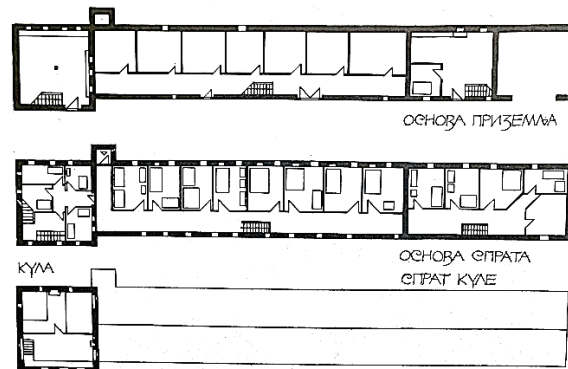
Fig. 8b Rangée de chambres à dormir à Đurakovac [alb. Gjurakoc] (d'après Branislav Kojić) ; dans B. Kojić, Seoska arhitektura i rurizam... , Belgrade, 1973, p. 74, fig. 116.
