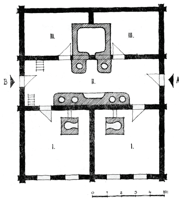
Fig. 20 Maison double du département de Poprad (d'après Jan Botík) ; 1 – chambre habitée ; 2 – chambre de passage ; 3 – cellier ; dans J. Botík, « Rodina... », p. 169, fig. 81.
