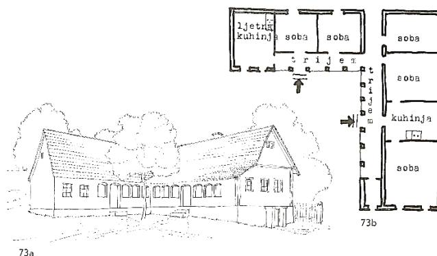
Fig. 17 Maison longue croate en forme de L, de Ožegovci (d'après Aleksandar Freudenreich) ; chambre à dormir ( soba ), cuisine ( kuhinja ), véranda ( trijem ) ; dans A. Freudenreich, Kako narod gradi , p. 53, fig. 73a et 73b.
