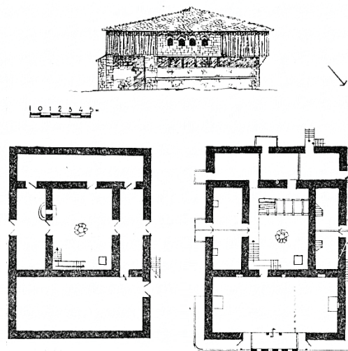
Fig. 9c Maison fortifiée à foyer central, et chambres à dormir, au village de Petit Shëngjin [alb. Shëngjini i Vogël] (d'après Ali Muka). Le plan de la grande maison (1), avec son foyer central ; dans A. Muka, « L'habitation rurale dans la Malessie... », p. 252, planche IX-2.
