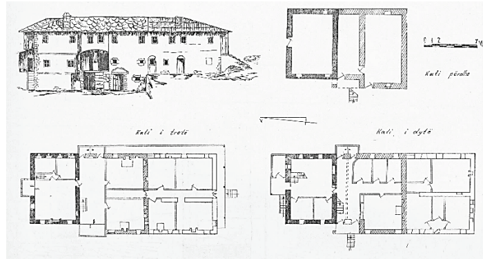
Fig. 5 Maison de Qarrishtë (Albanie), construite en trois étapes (d'après Ali Muka). En haut, le plan du rez-de-chaussée ; en bas, à droite, le deuxième niveau, à gauche le troisième ; dans A. Muka, « Constructions dans les environs de Librazhd », Ethnographie albanaise 10, 1980, p. 221, planche VI.
