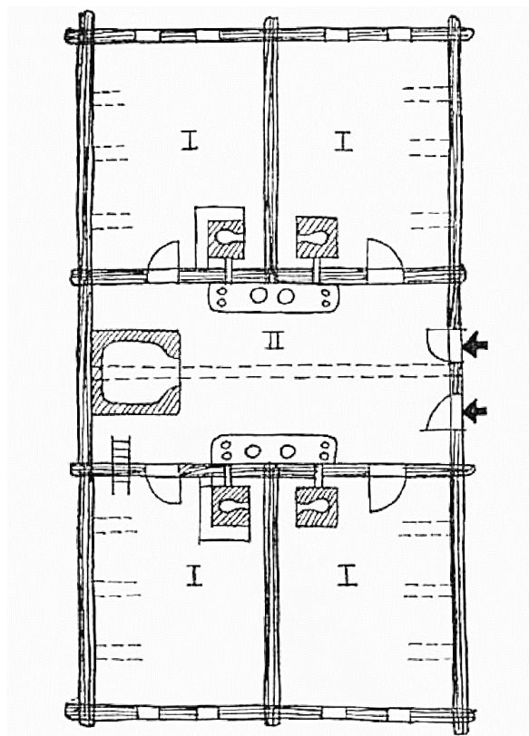
Fig. 21 Maison double de la Slovaquie du Nord – Štôla (d'après Soňa Švecová) ; dans S. Švecová, « Die Beziehungen zwischen Architektur und Familien Organisation in der Slowakei », Deutsches Jahrbuch für Volkskunde (Berlin) 13, première partie, 1967, p. 98, fig. 5.
