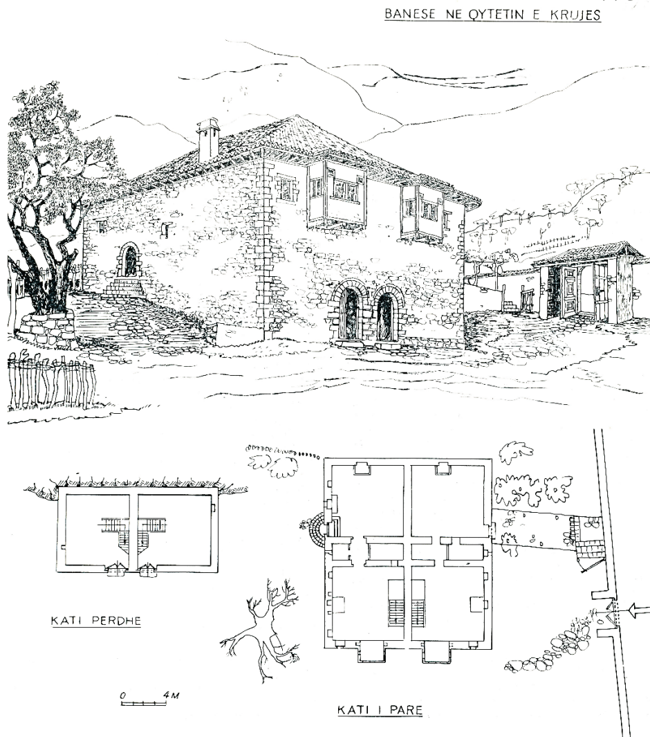
Fig. 2 Maison double de Kruja, Albanie (d'après Emin Riza) ; dans E. Riza, « Banesa dyfamiare në qytet », Monumentet 2, 1981, p. 115-125, p. 123, planche V, maison n° 8.
